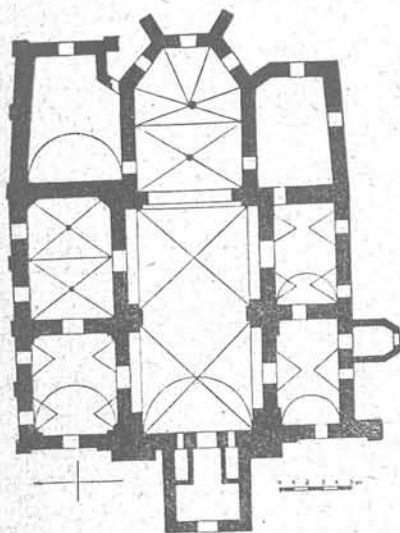
Pila — plan kościoła św. Jana.
