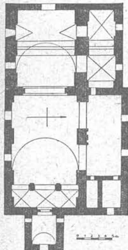
Pillica — plan kościoła OO. Reformatów.
