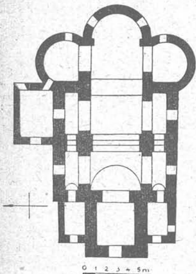
Skarżyce — plan kościoła.
