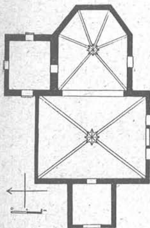
Wolbrom — plan kościoła drewnianego.
